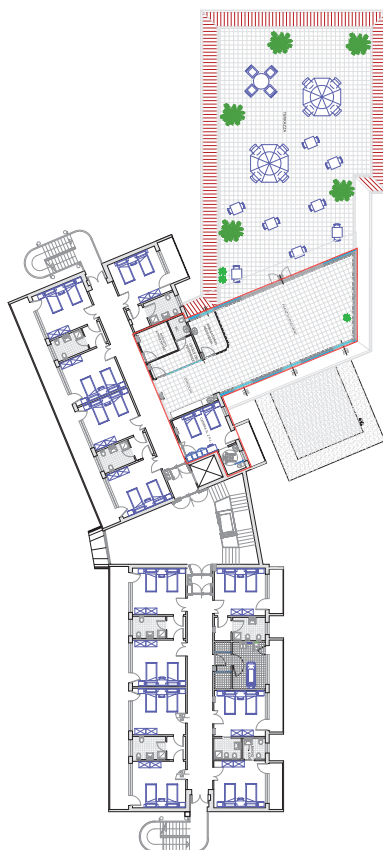
Progetto di ampliamento pianta 2° piano
